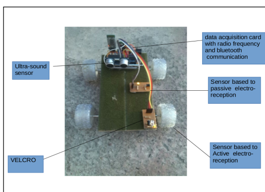
Figura 1. Vehículo motorizado FREEinfrarOSI. Autor (2017).
